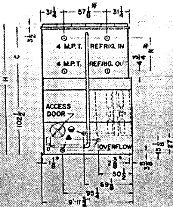
VIEW A-A
