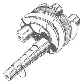
DISCHARGE
